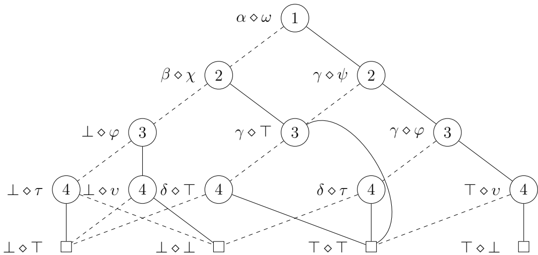
Figuur 1: Voorbeeld: twee BDD s die samengesmolten worden door gebruik te maken van formule 1. Let er wel op dat dit voorbeeld geen ontbrekende laag van knopen heeft, waardoor knopen van alle niveaus beschikbaar zijn. Op het moment dat de \diamond ingevuld gaat worden is het ook zaak om de bladeren (zie vergelijking 2) te vereenvoudigen
