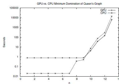
Figuur 5: Uitvoertijden (logaritmische schaal) van de CPU en GPU gebaseerde minimale dominantie implementaties welke y(Q_n) uitrekenen. Hoe groter n wordt des te beter de GPU gaat presteren in vergelijking met de CPU .
